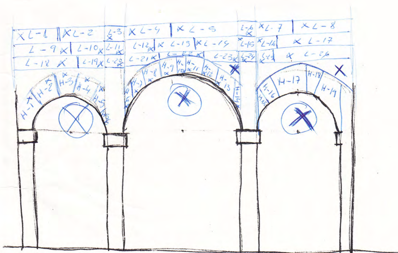
FACHADA LATERAL DERECHA (VISTA INTERIOR)
