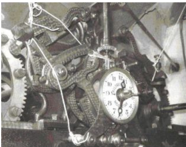
Maquinaria actual del reloj del campanario.
